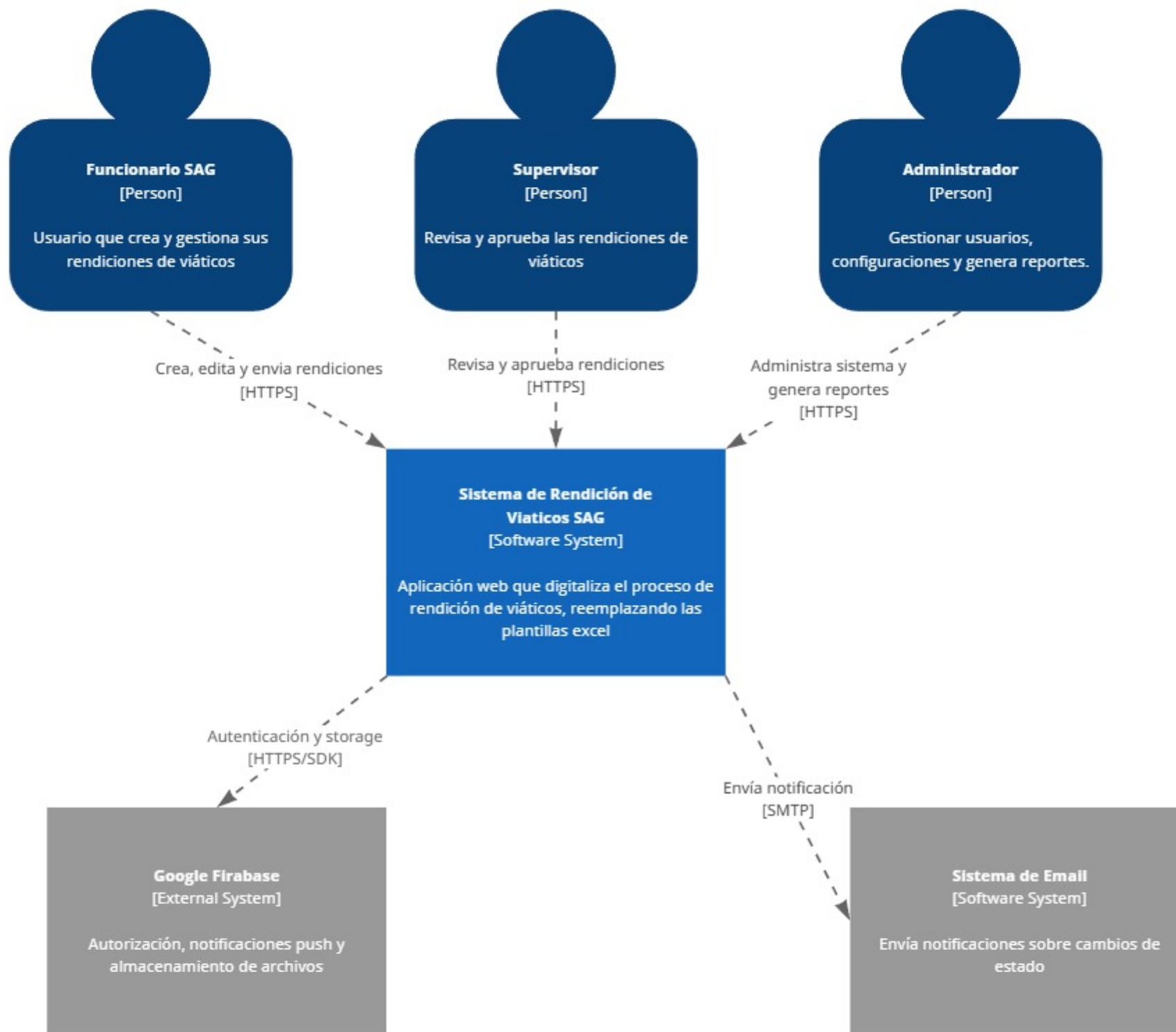
Diagrama de contexto del Sistema de Rendición de Viaticos Sag
